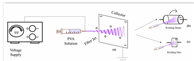
Gambar 2.5. Ilustrasi Sistem Electrospinning untuk Fabrikasi Nanofiber PVA [12]
